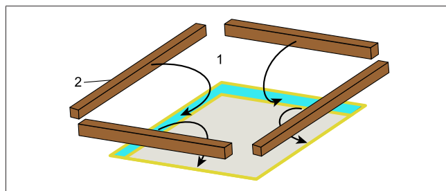
Abb. 9 Dachverstärkung
