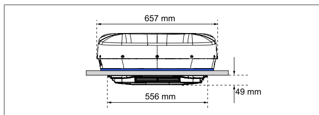
Abb. 8 Einbaumaße (Ansicht von vorn)
