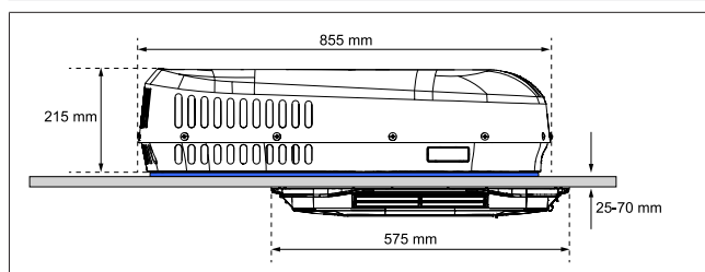
Abb. 7 Einbaumaße (Seitenansicht)
