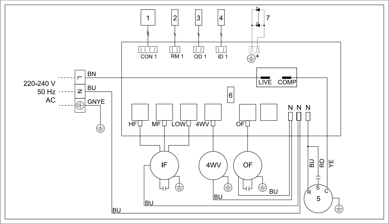
Abb. 58 Schaltplan
