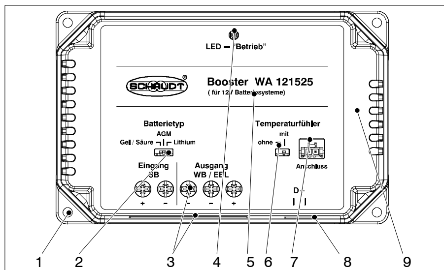
Bild 8 Aufbau Booster WA 121525
