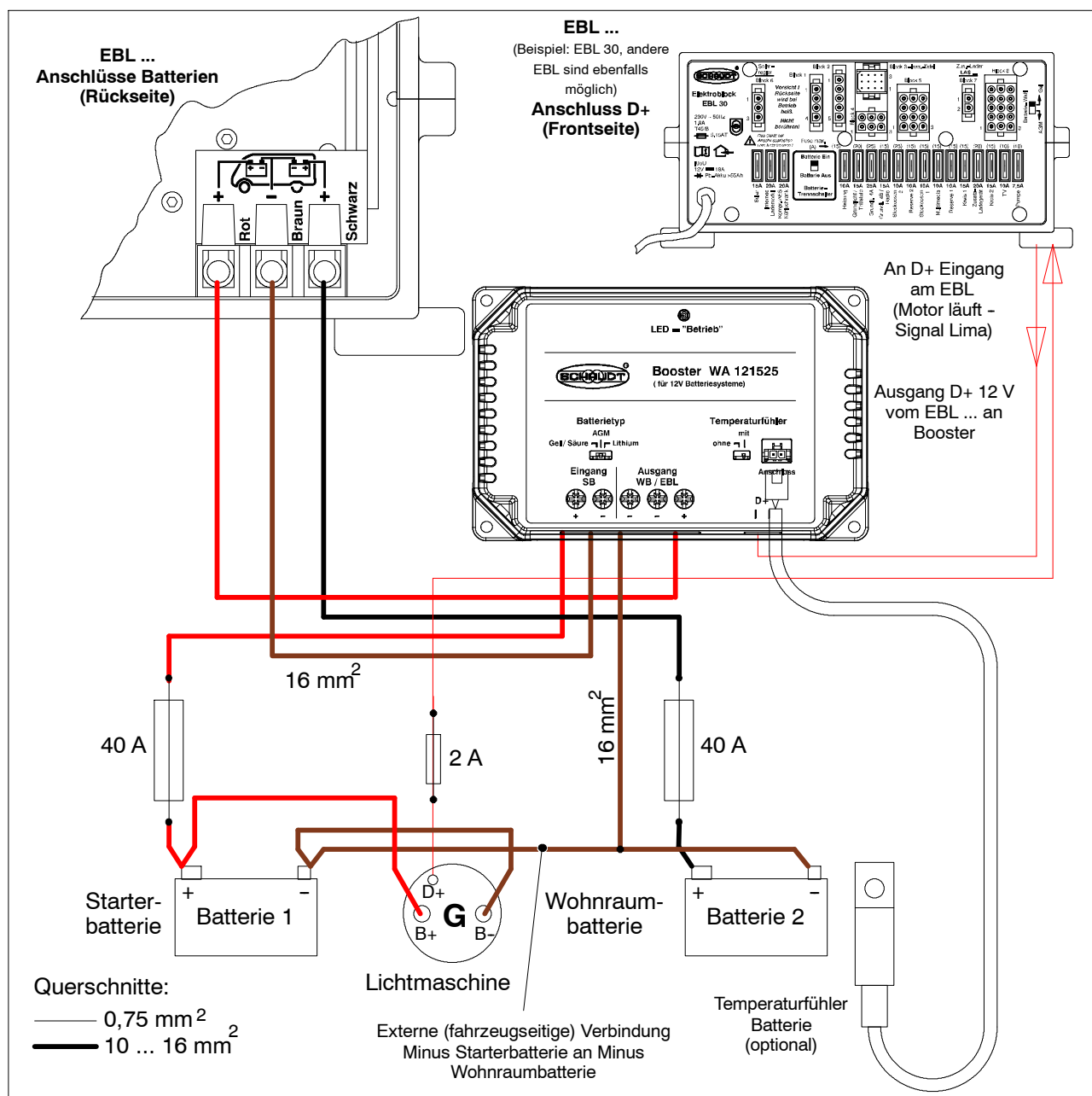
Bild 3 Fahrzeuge mit Schaudt EBL ... - externe Masseverbindung
