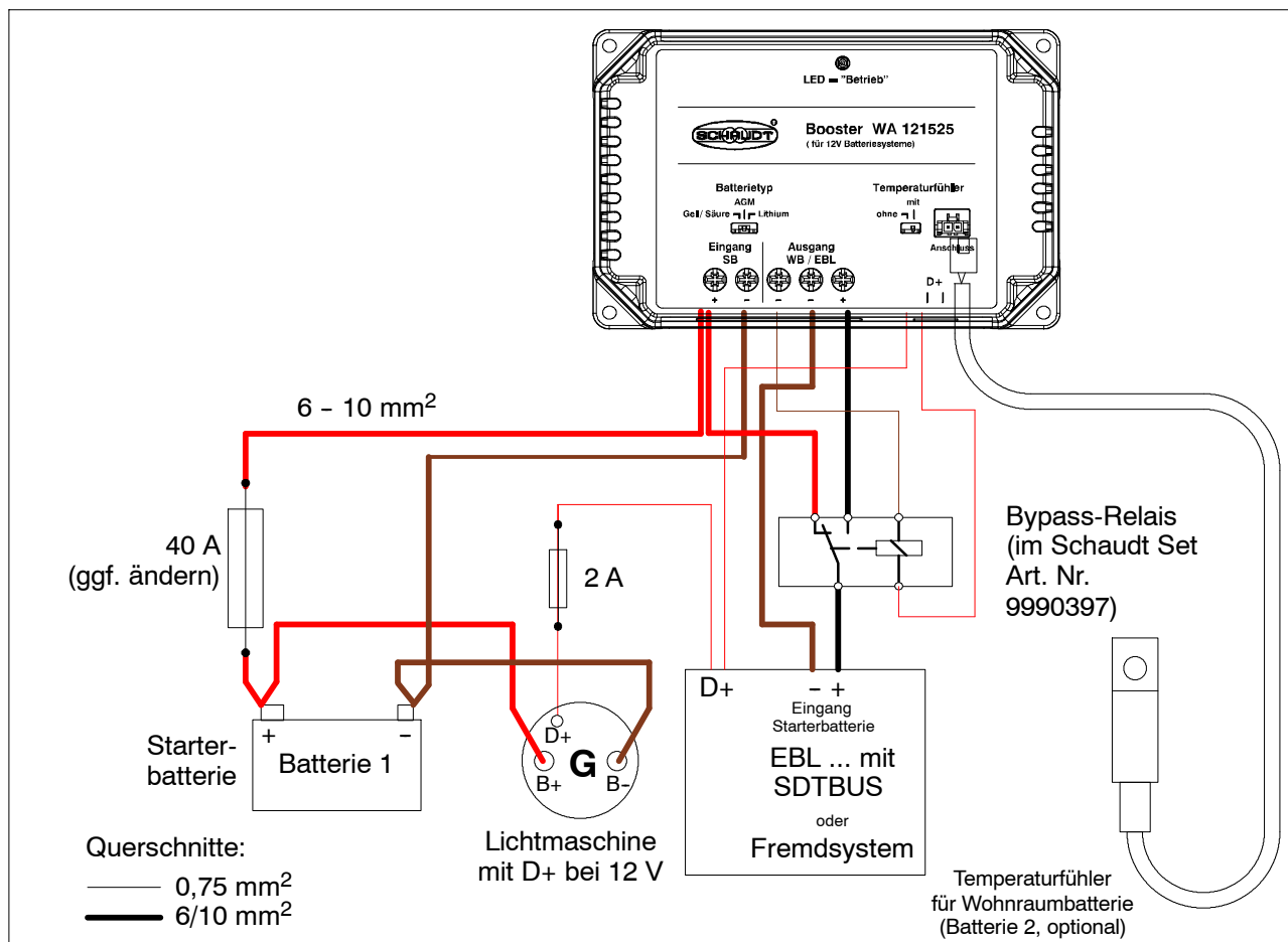
Bild 5 Fahrzeuge mit SDTBUS-Systemen oder Stromversorgungen ohne Schaudt EBL ...
