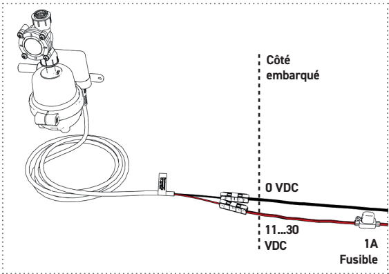
Figure 15 : Raccordements électriques
